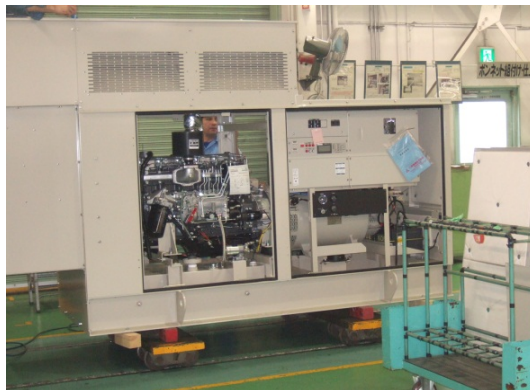
三菱パッケージ発電機 PG-Q シリーズ
