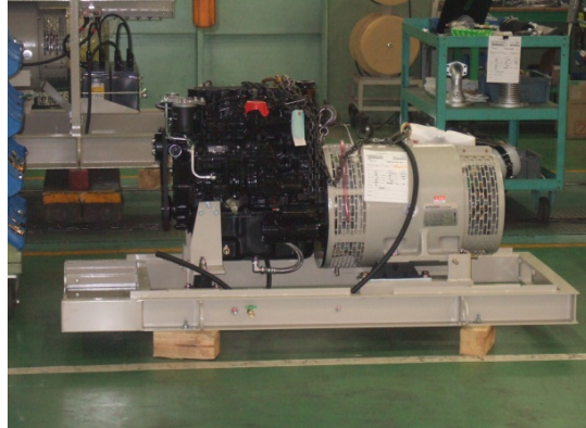
三菱パッケージ発電機 PG-Q(発電機)
